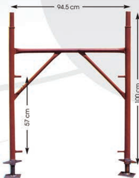
ΠΛΑΙΣΙΟ ΕΞΩΤΕΡΙΚΗΣ ΟΨΕΩΣ (ΚΩΔ. P 09 ) με σωλήνα \Phi 48 2 mm ET και 3 mm BT
