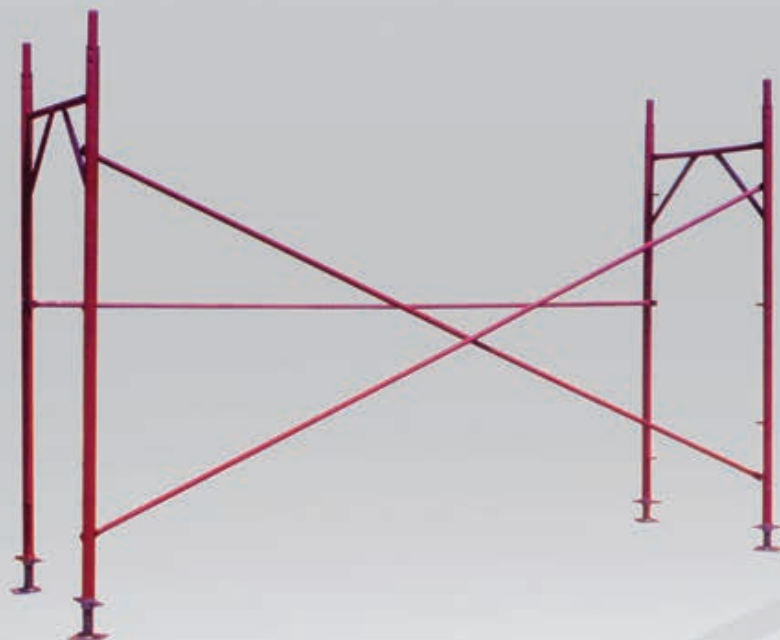
ΠΥΡΓΟΣ ΕΞΩΤΕΡΙΚΗΣ ΟΨΕΩΣ (ΚΩΔ. P 30 ) παλαιού τύπου με χιαστό και κουπαστή διαστάσεις 200x350 cm
