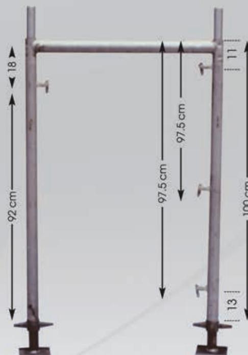
ΠΛΑΙΣΙΟ ΕΞΩΤΕΡΙΚΗΣ ΟΨΕΩΣ Γερμανικής (ΚΩΔ. P 10 ) προδιαγραφών ΒΤ με σωλήνα \Phi 48
