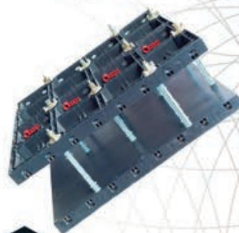
Πλαστικότυποι τοιχείων (ΚΩΔ. P 73)
