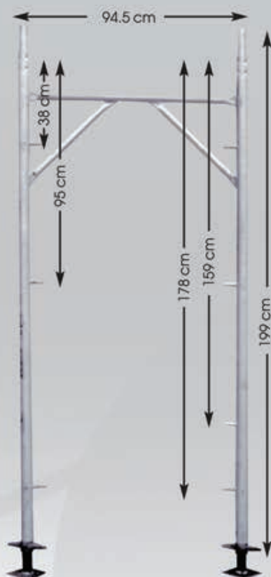
ΠΛΑΙΣΙΟ ΕΞΩΤΕΡΙΚΗΣ ΟΨΕΩΣ (ΚΩΔ. P 07 ) με σωλήνα \Phi 48 2 mm και 3 mm BT
